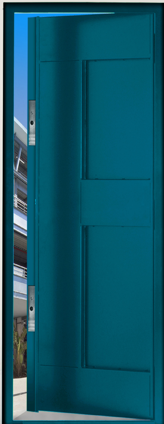
Modèle bloc-porte présenté avec 4 omégas et 2 ventouses 300 kg
