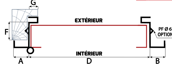
Croquis 1 VANTAIL poussant pour format 1000 x 2300 mm (au-delà options)
