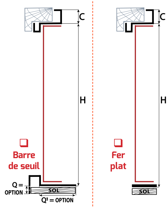
Croquis 1 VANTAIL poussant pour format 1000 x 2300 mm (au-delà options)
