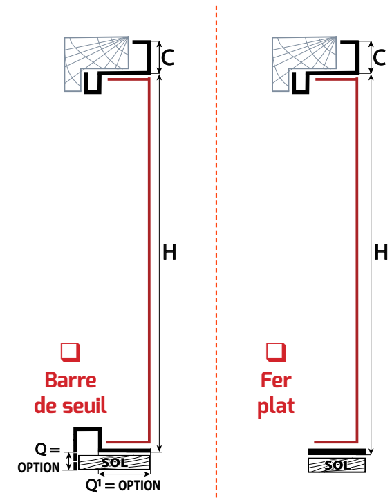
Croquis 1 VANTAIL poussant pour format 1000 x 2300 mm (au-delà options)
